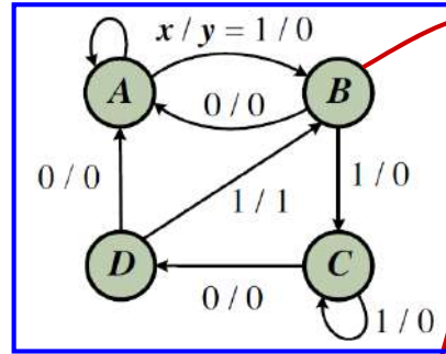
Περιγραφή μοντέλου Mealy
